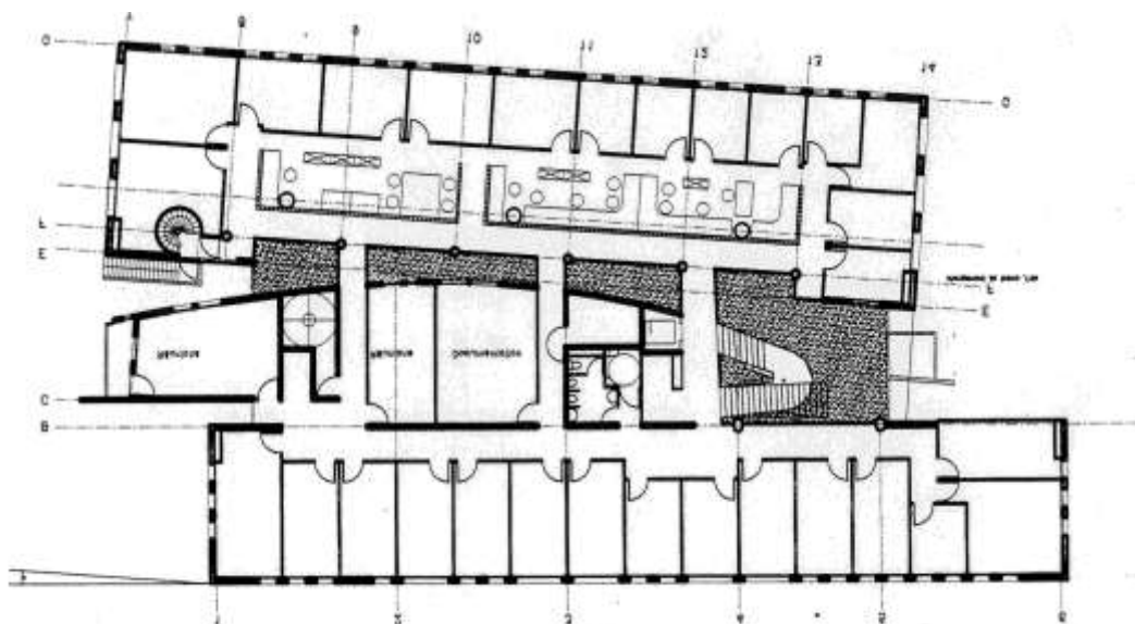
combi – office (Projet Cemagref ; architectes Quatre Plus)
